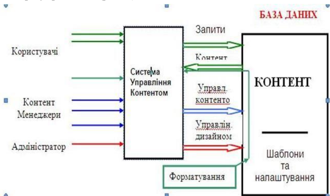
Рис.1. Основні функції систем управління Web-контентом [9]
